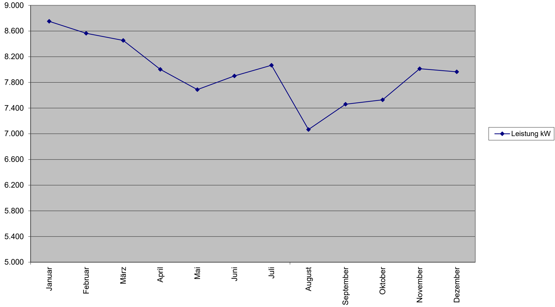
Lastverlauf Netz Budenheim 2023
