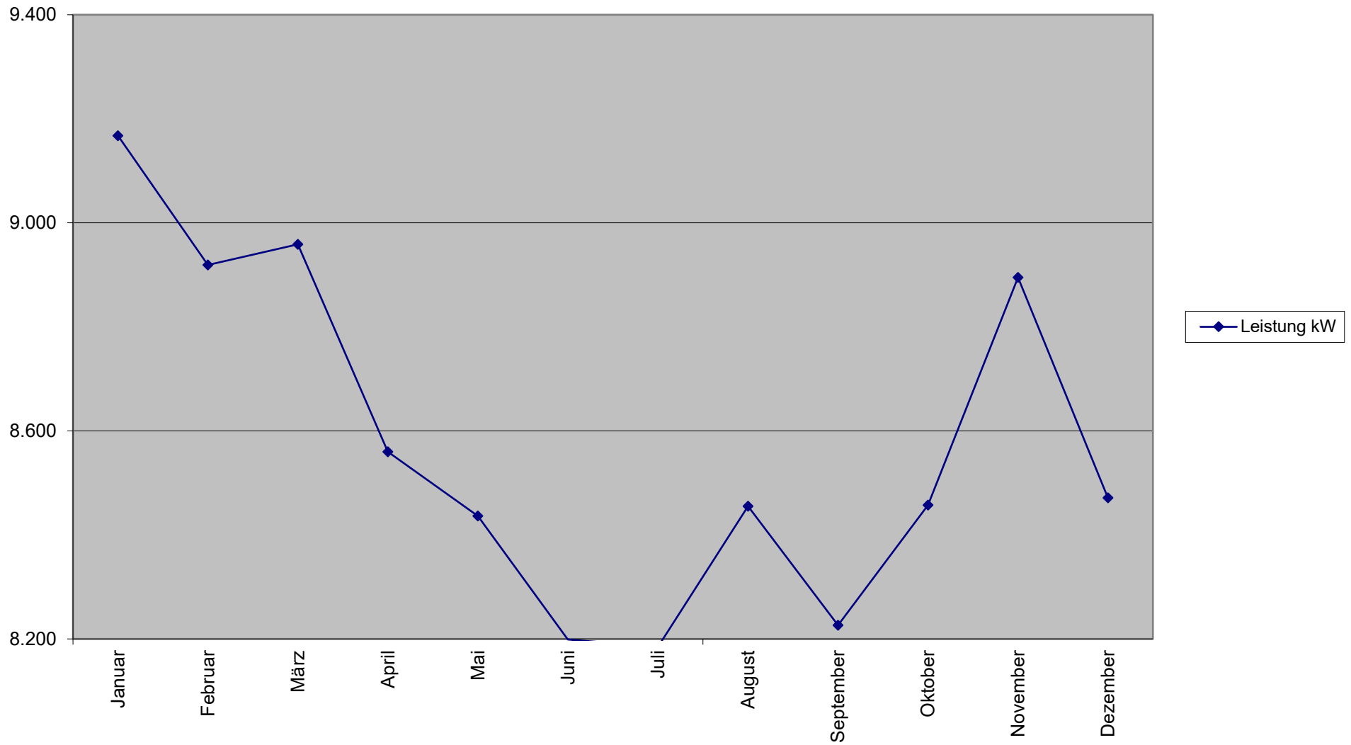
Lastverlauf Netz Budenheim 2020
